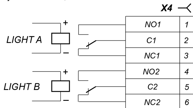
Рисунок 16. Выходные каскады для Light A и Light B
